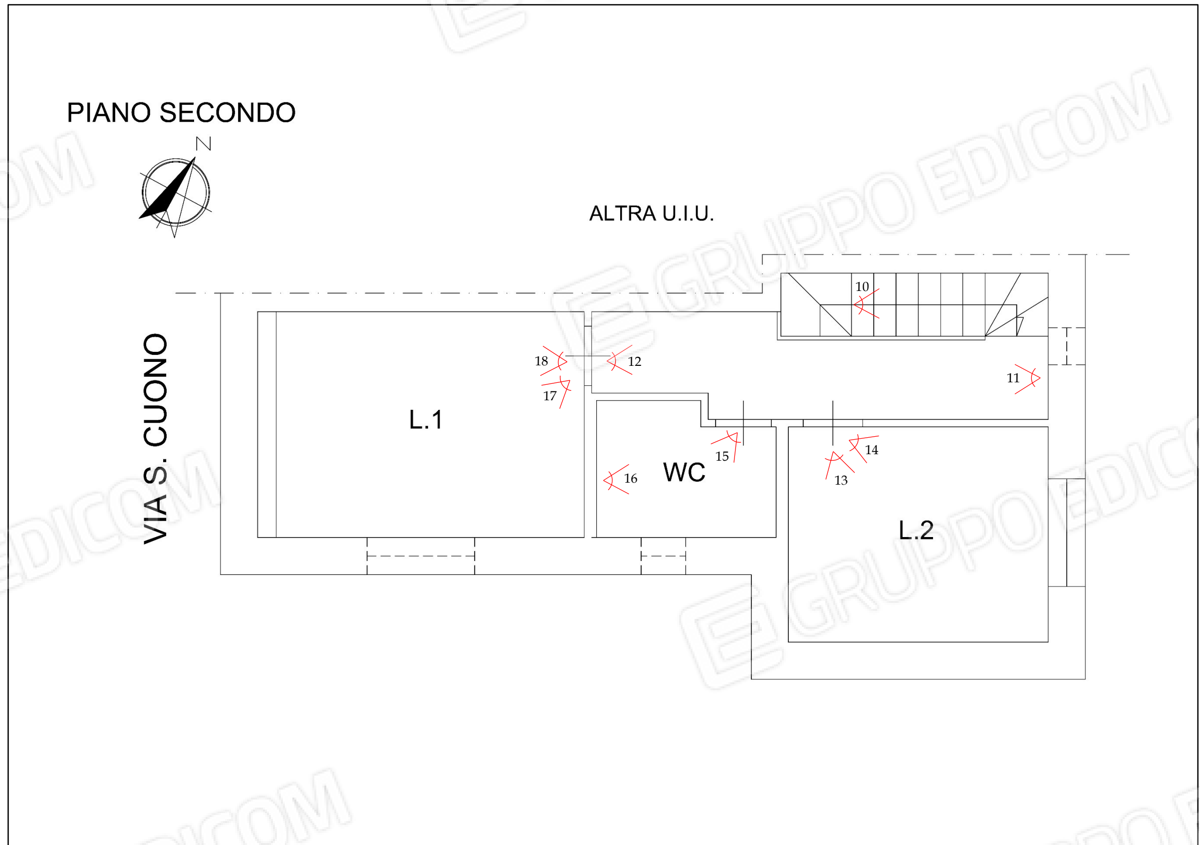
Figura 2: Planimetria di rilievo con indicazione dei coni ottici (piano secondo)
